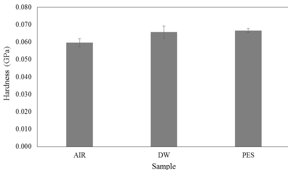
Slika3. Tvrdća dobijena nanoindentaciom ispitivanih uzorka za bazu proteze izloženih vazduhu (AIR), destilovanoj vodi (DW) i rastvoru ekstrakta lista morača (PES)
